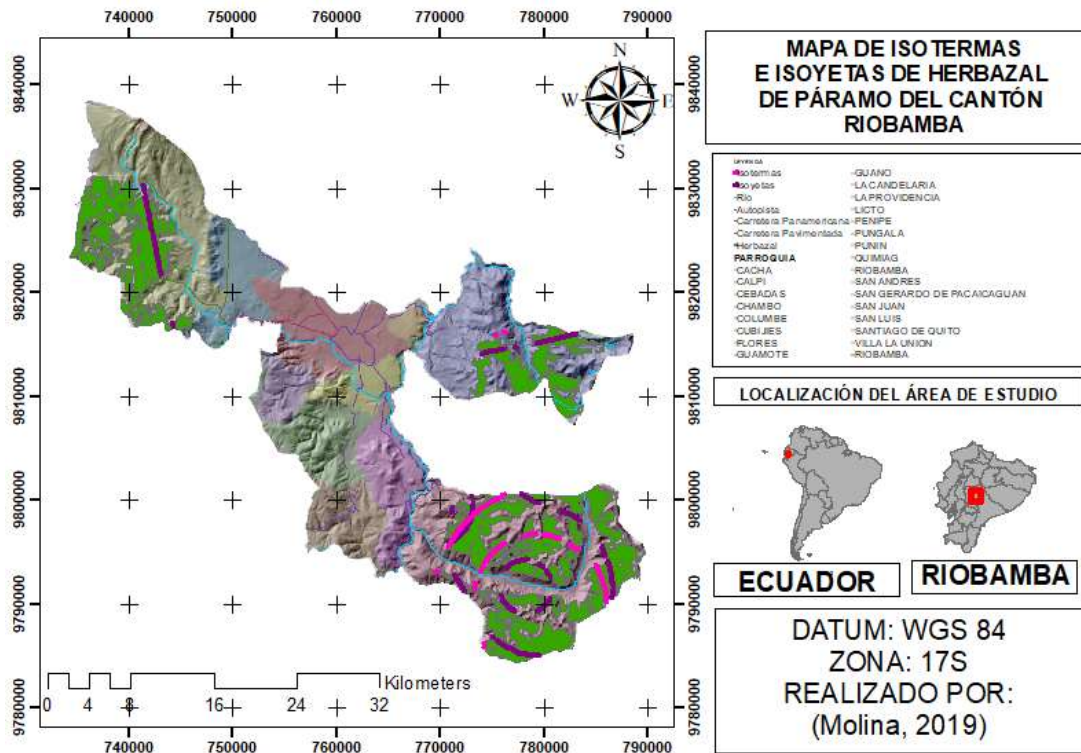
Figura 7. 5. Isoyetas e isoterms de la formación herbazal del páramo en el cantón Riobamba
