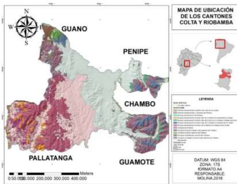
Figura 6. 1. Ubicación geográfica de los cantones Colta y Riobamba de la provincia de Chimborazo
