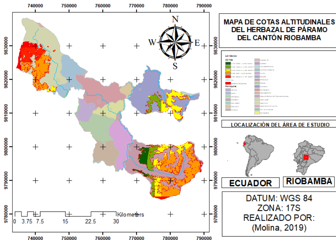
Figura 7. 2. Cotras altitudinales de la formación herbazal de páramo en el cantón Riobamba Nota: (Molina, 2019).
