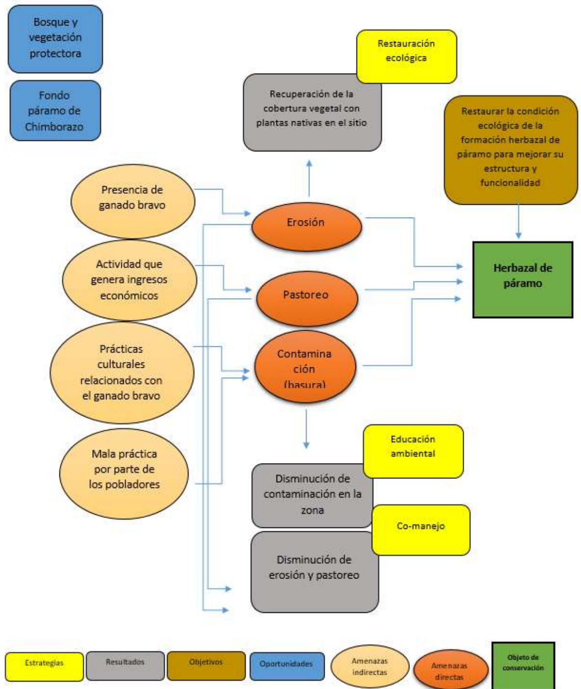
Figura 7. 51. Estructuración de lineamientos de la formación herbazal de páramo del cantón Colta Nota: (Molina, 2019)
