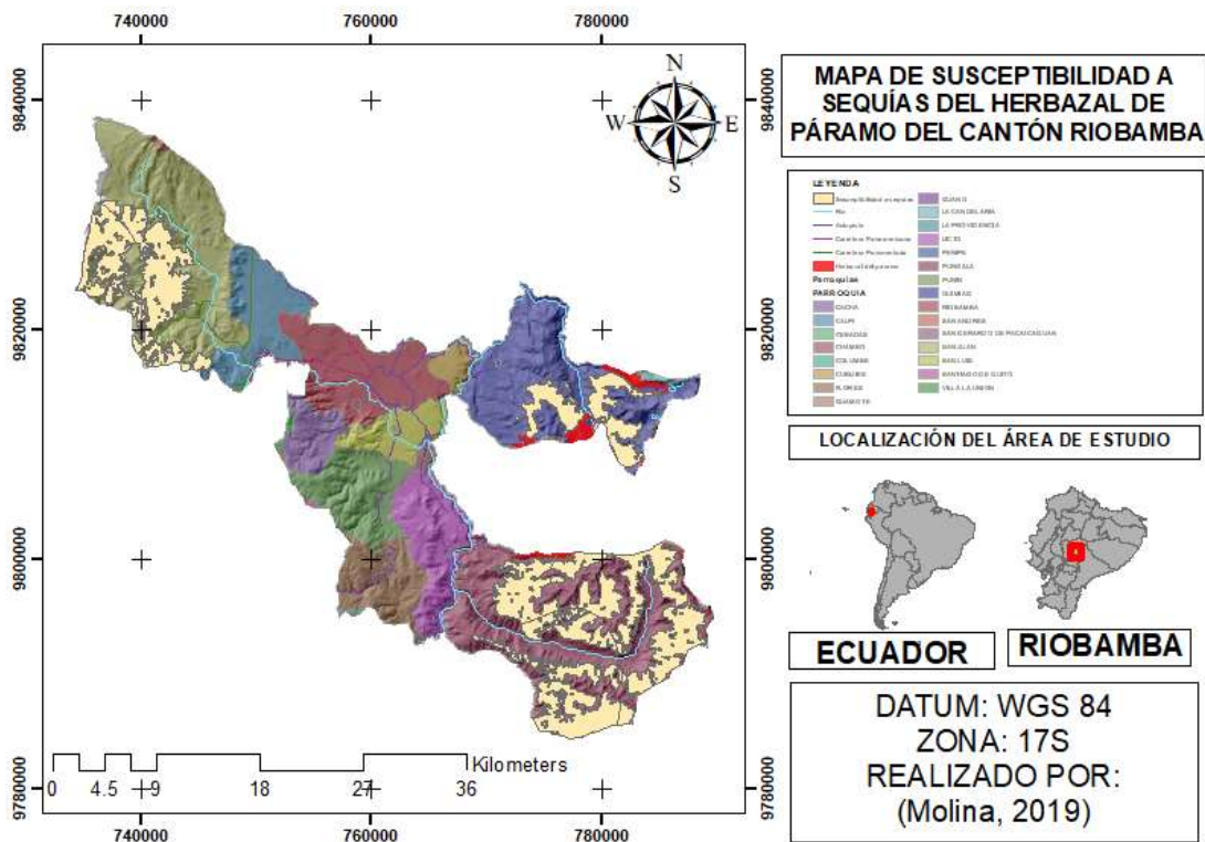
Figura 7. 8 Susceptibilidades a sequías en la formación herbazal de páramo en el cantón Riobamba. Nota: (Molina, 2019).
