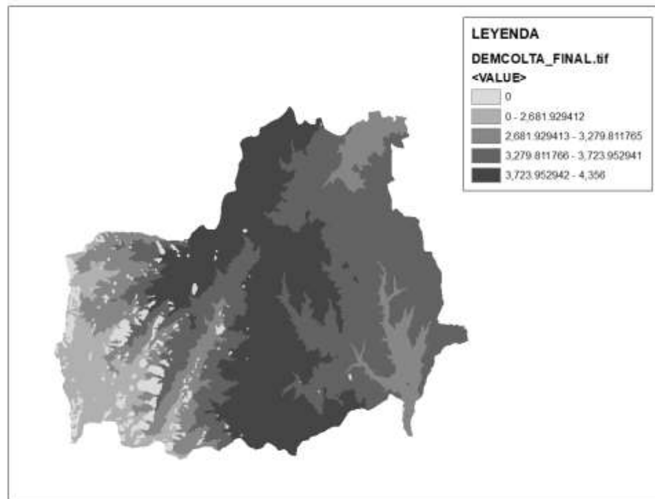
Figura 7. 45. Modelo de elevación digital del cantón Colta. Nota: (Molina, 2019).
