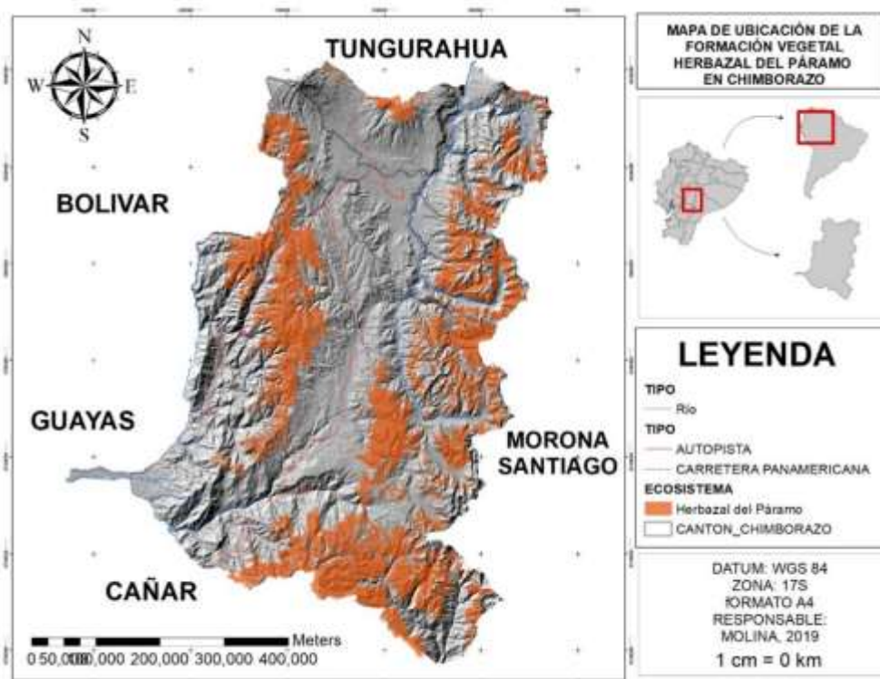
Figura 5. 1. Ubicación geográfica del herbazal del páramo en la provincia de Chimborazo.
