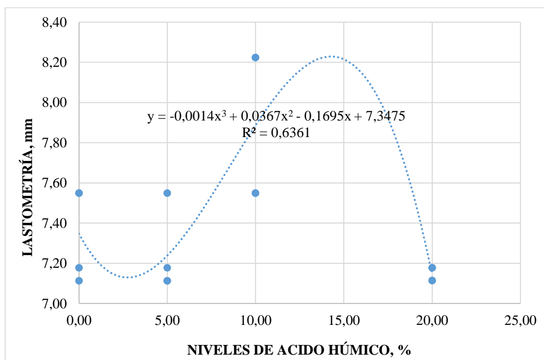
Gráfico 5-4: Regresión del porcentaje de elongación de los cueros caprinos curtidos por efecto de la adición de diferentes niveles de ácido húmico en combinación con tara
